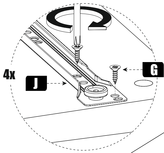
Шуруп 4x13
